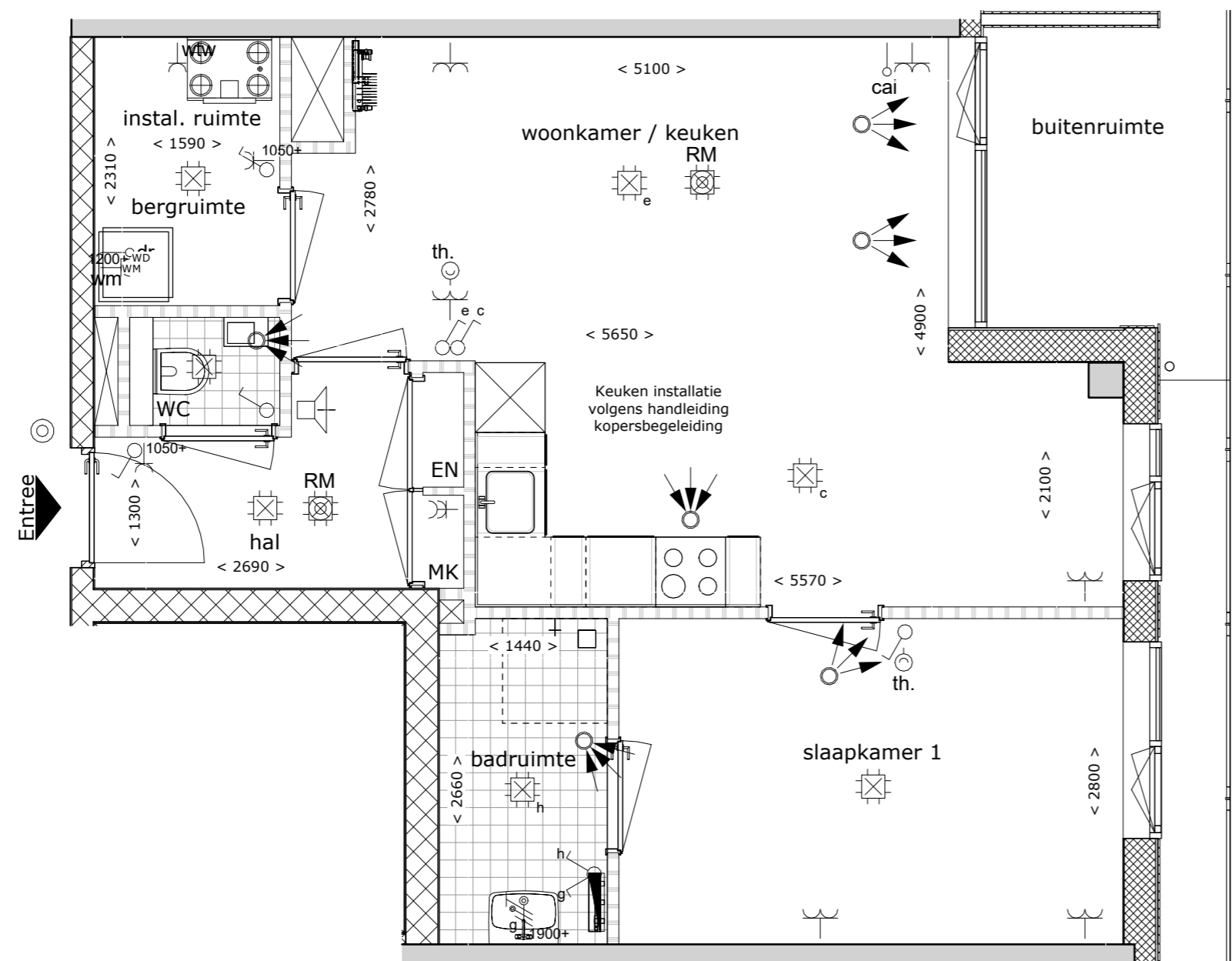
Bouwnummer A014 1 : 50
