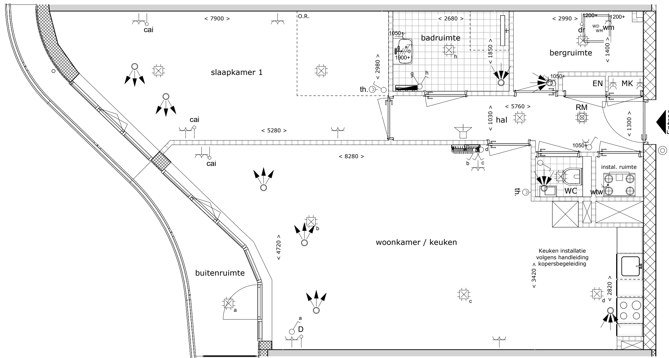
Bouwnummer A017 1 : 50
