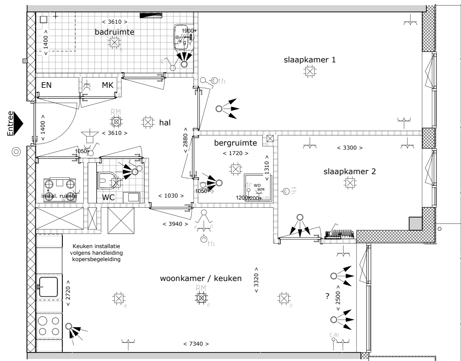
Bouwnummer A023 1 : 50
