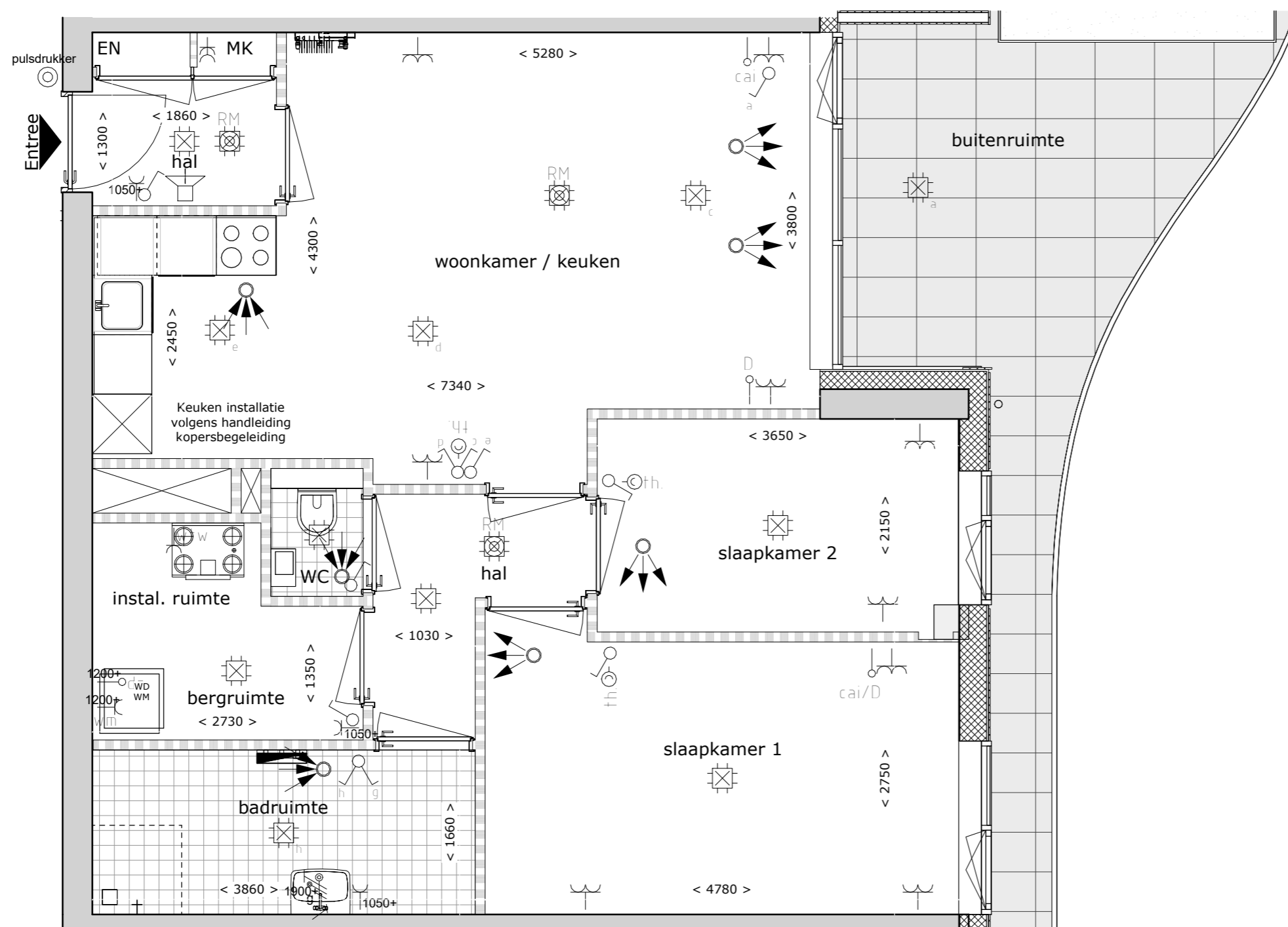
Bouwnummer A003 1 : 50
