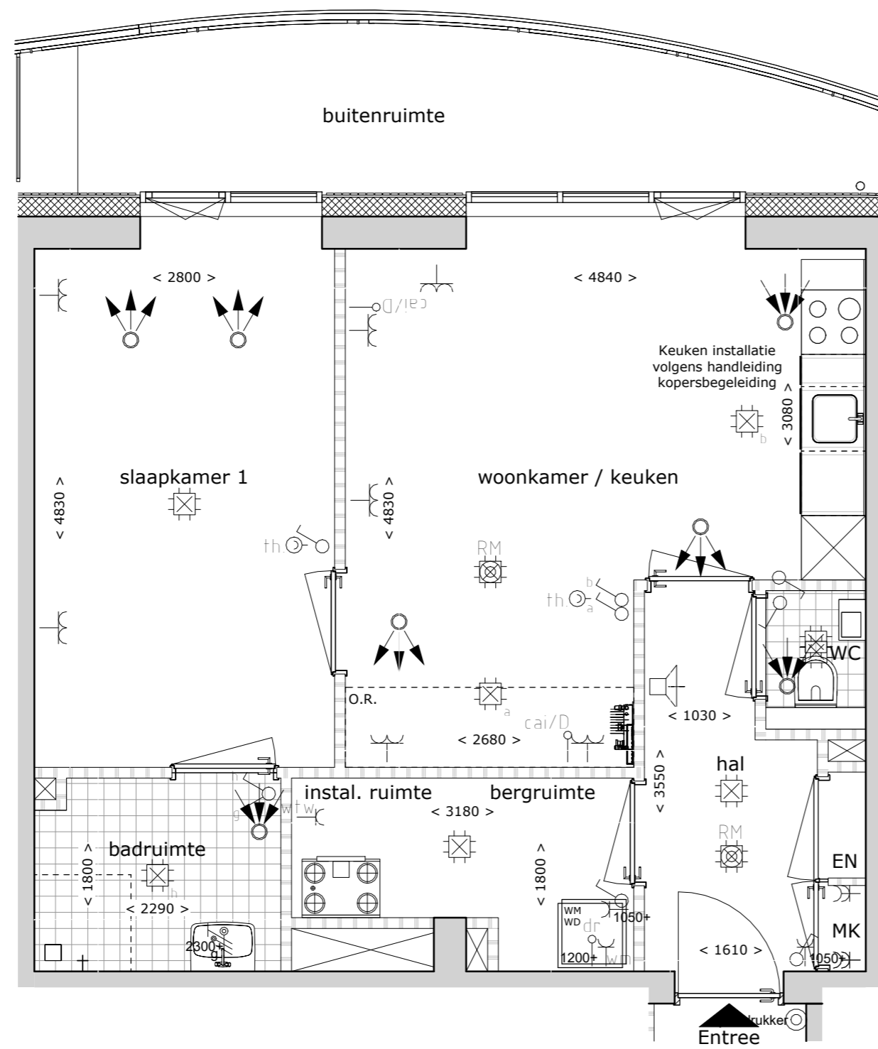
Bouwnummer A040 1 : 50
