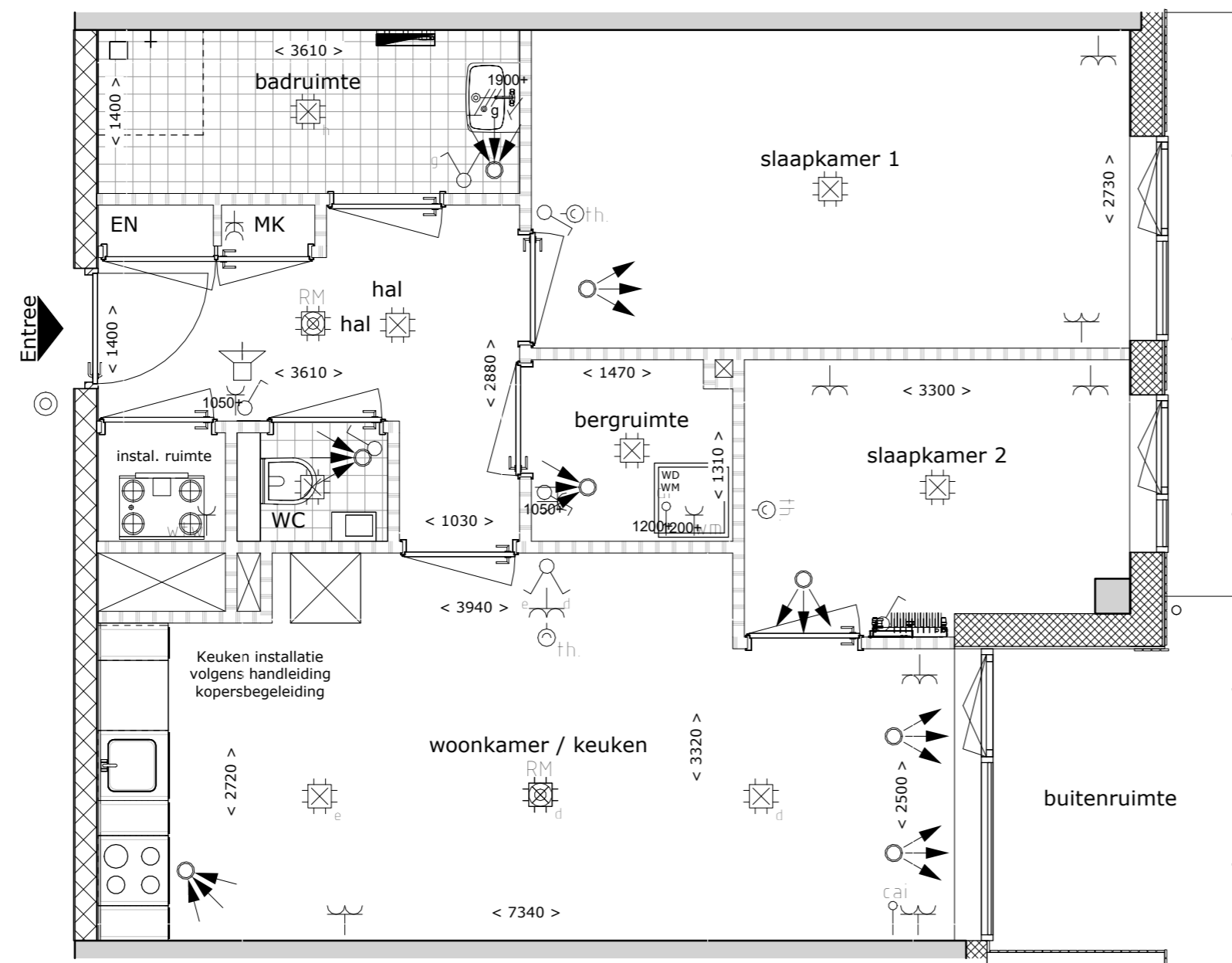
Bouwnummer A043 1 : 50
