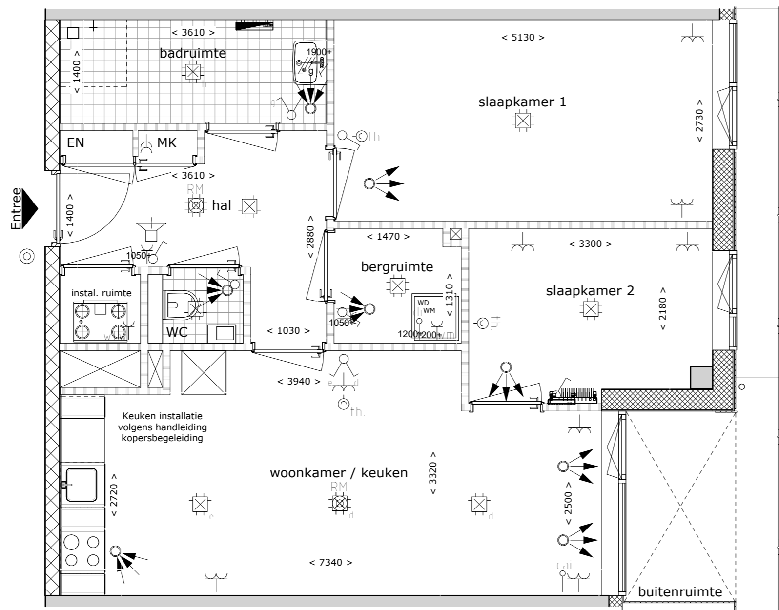
Bouwnummer A053 1 : 50
