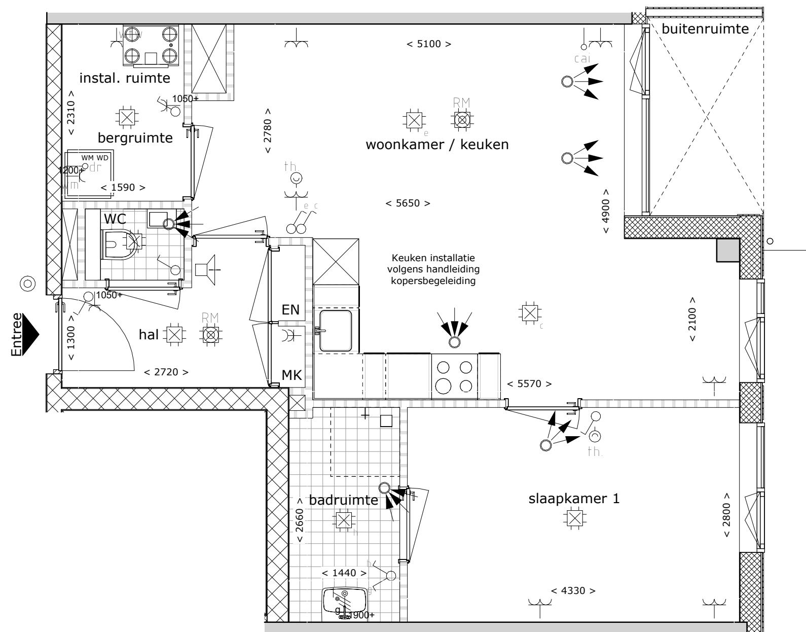
Bouwnummer A054 1 : 50
