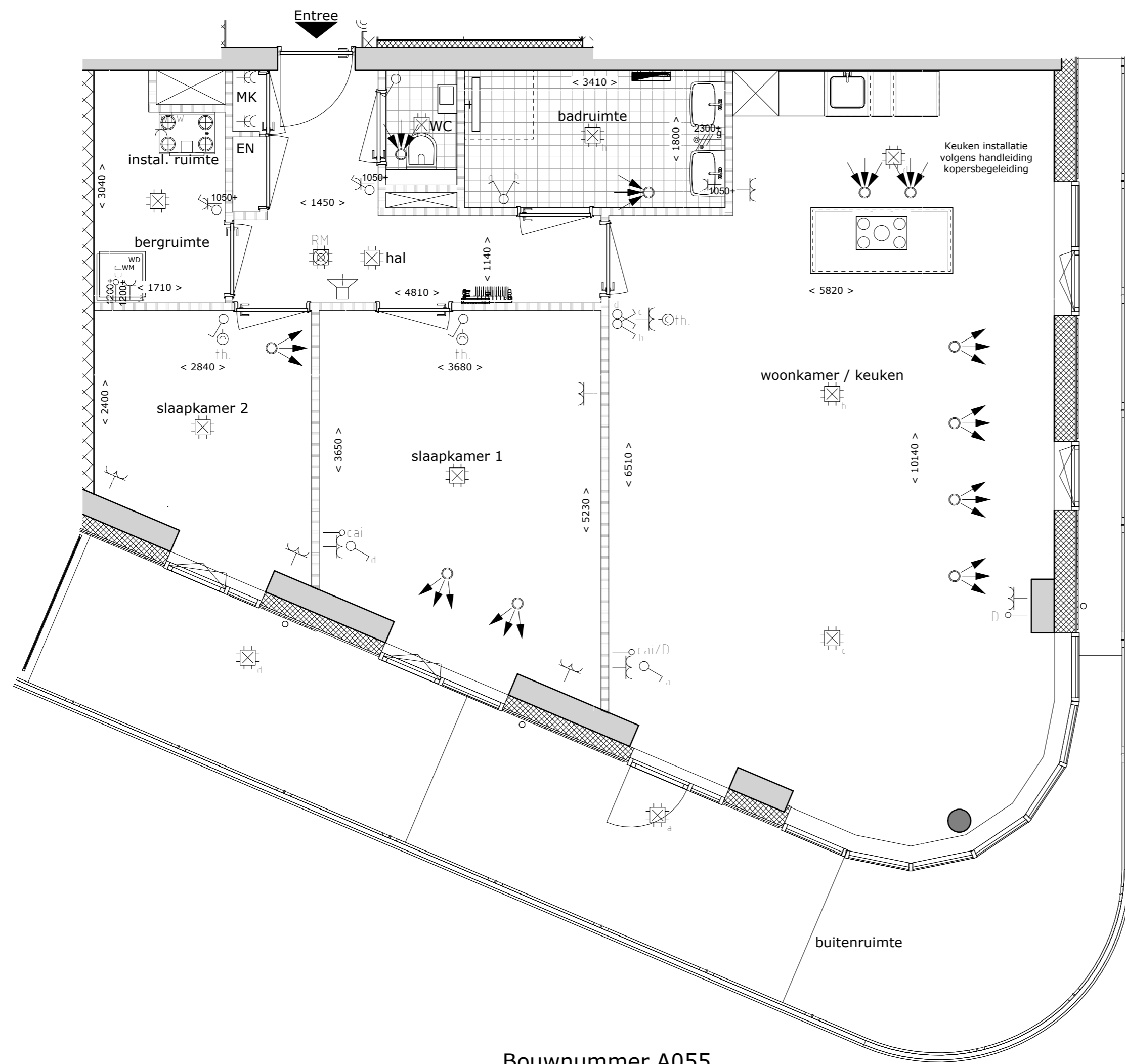
Bouwnummer A055 1 : 50
