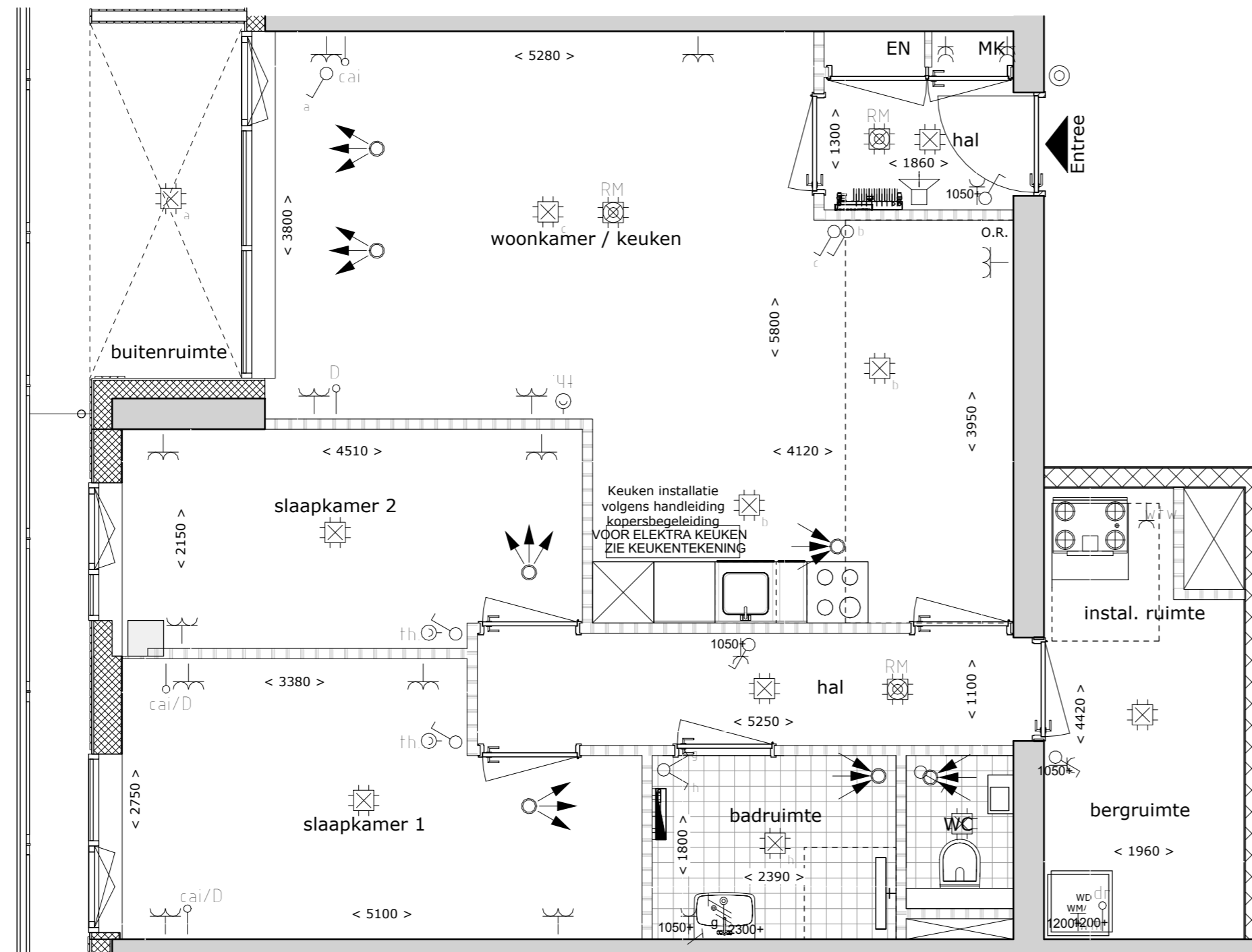
Bouwnummer A058 1 : 50
