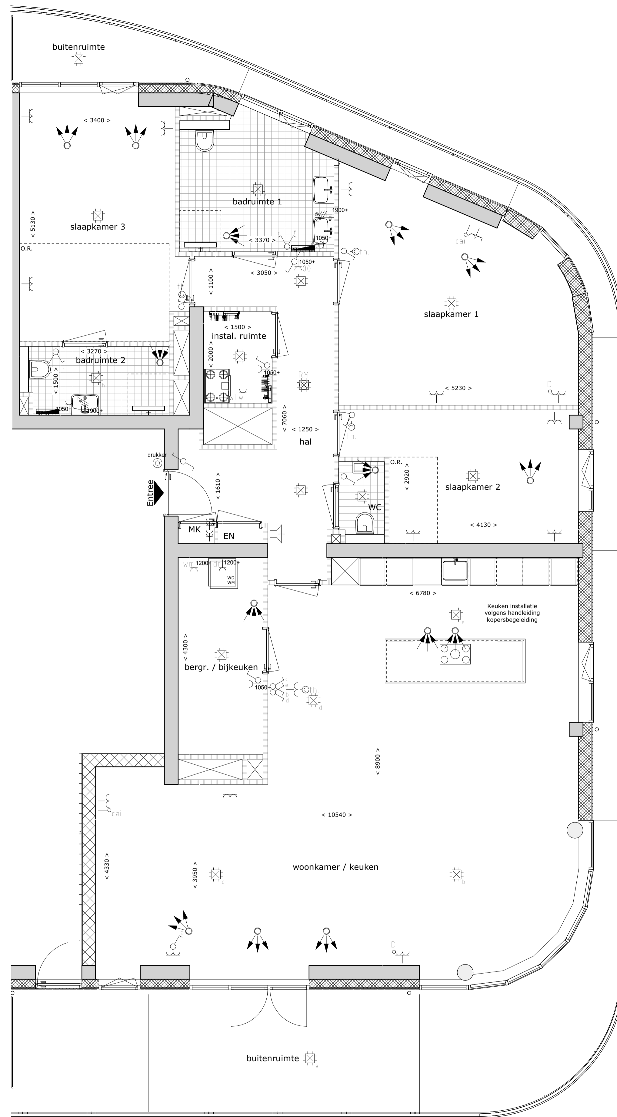
Bouwnummer A064 1 : 50
