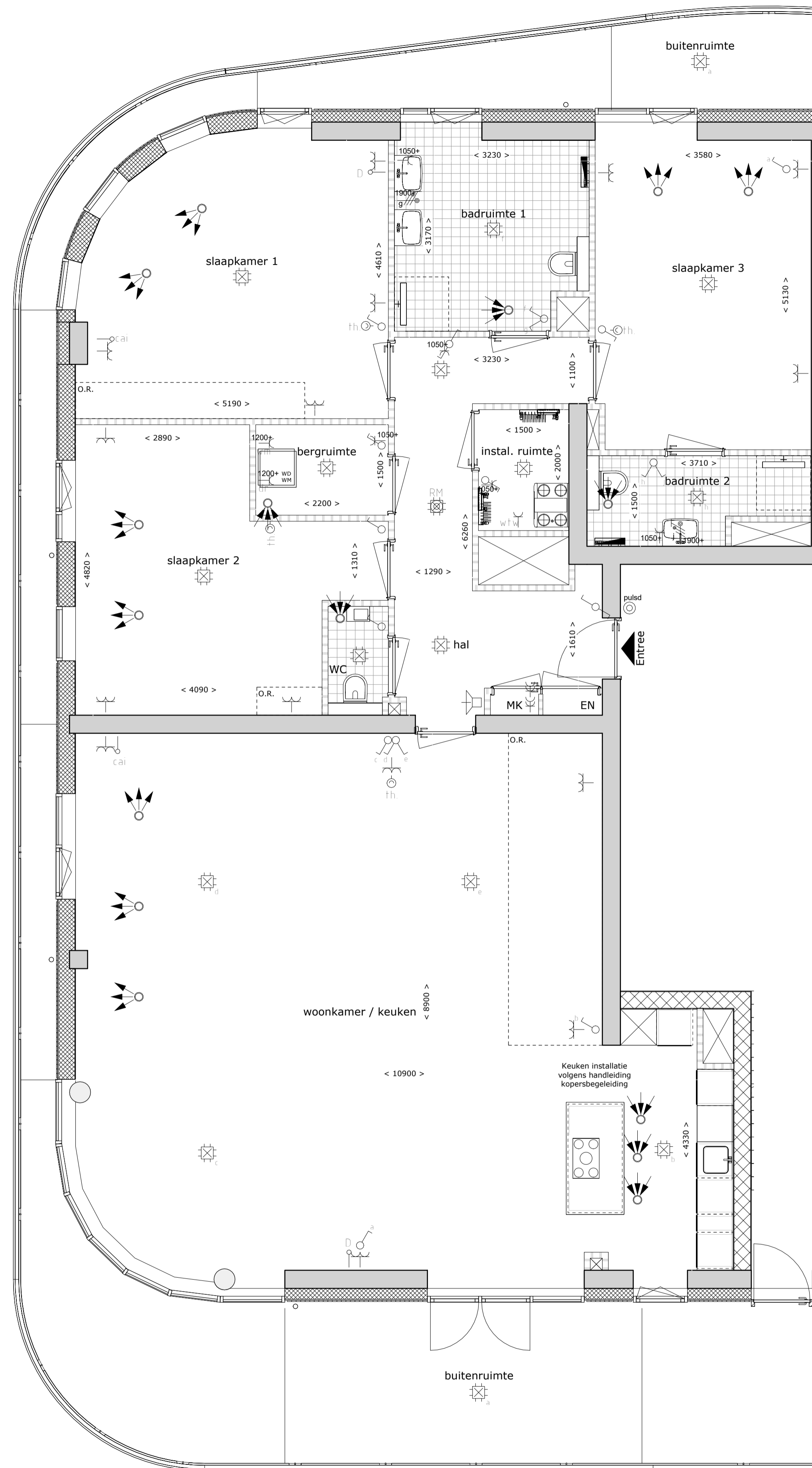
Bouwnummer A065 1 : 50
